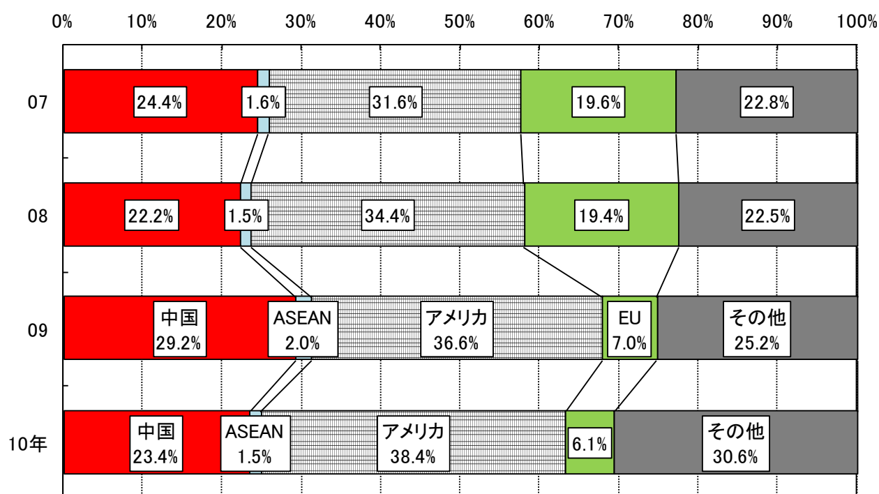
図表3-1-6 九州の自動車の輸出国地域別構成比の推移
