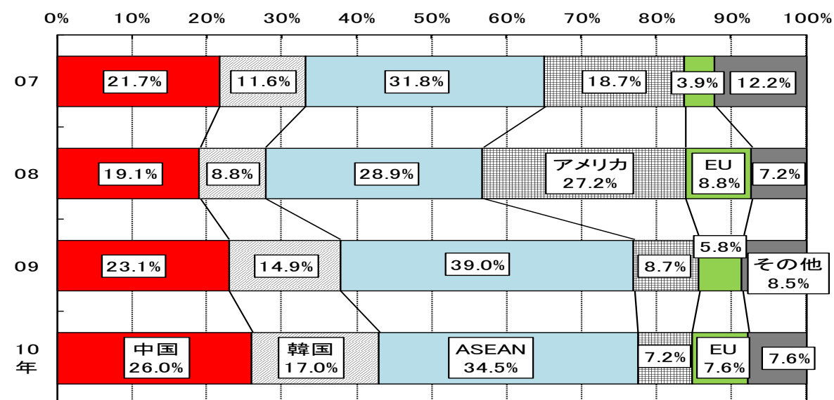
図表3-1-9 九州の自動車部品の輸入国地域別構成比の推移
