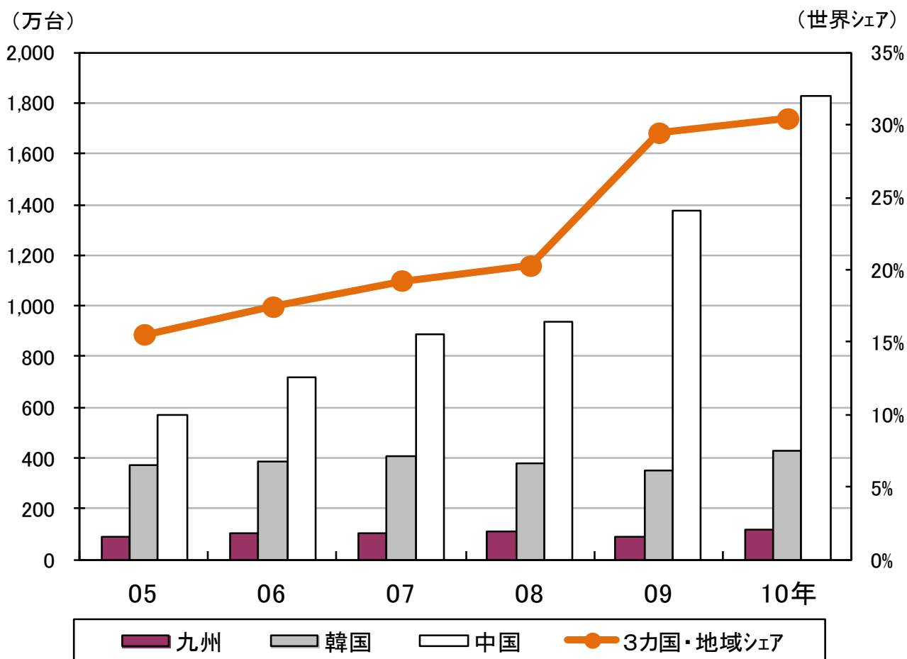
図表3-1-3 九州・韓国・中国の自動車生産台数の推移
