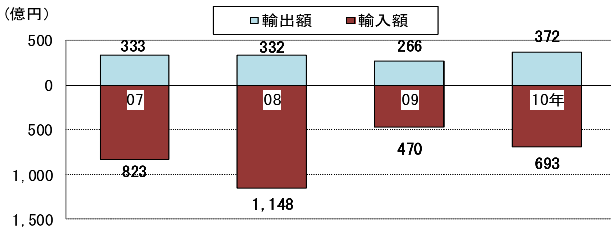
図表3-1-8 九州の自動車部品の輸出国地域別構成比の推移
