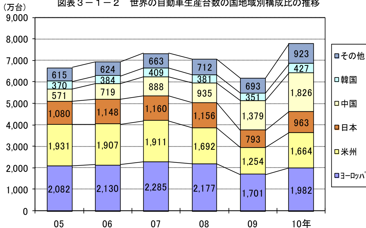
図表3-1-2 世界の自動車生産台数の国地域別構成比の推移
