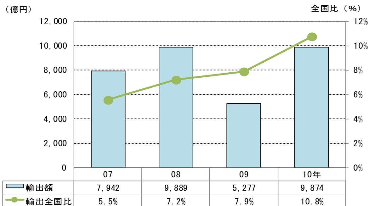
図表3-1-5 九州の自動車の輸出額推移
